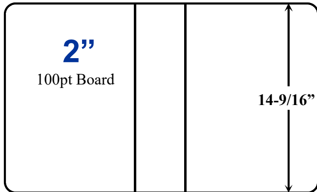
D-R SD Ring 11-1/4" 3-1/16" 11-1/4" Die # LB334
