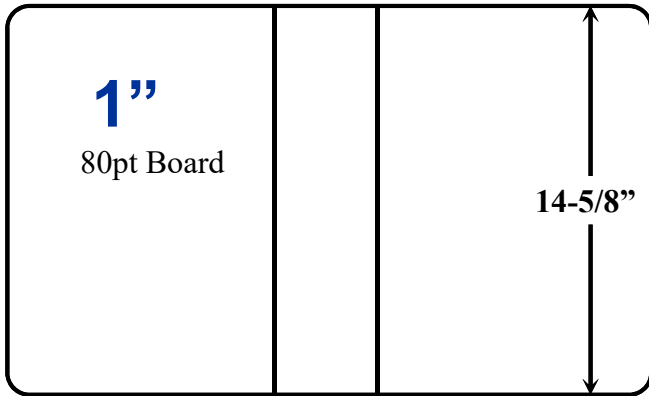
D-R SD Ring 10" 1-11/16" 10" Die # LB70
