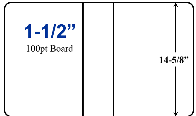
D-R SD Ring 10-11/16" 2-3/16" 10-11/16" Die # LB231
